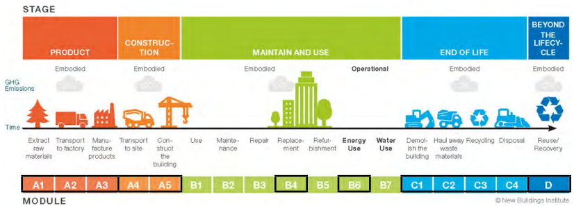
Figura 13. El ciclo de la vida del edificio. Tomado de Lifecycle stages of building carbon. Data source: BS EN 15978:2011 - Source: Bowles, Cheslak and Edelson.
