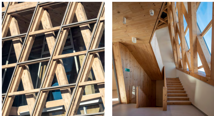
Figura 10: Celosías de fachada. Celosía sur, detalle desde el exterior (izq.), y celosía norte, aspecto desde el interior (dcha.). Fotografías: Héctor Santos-Díez.
