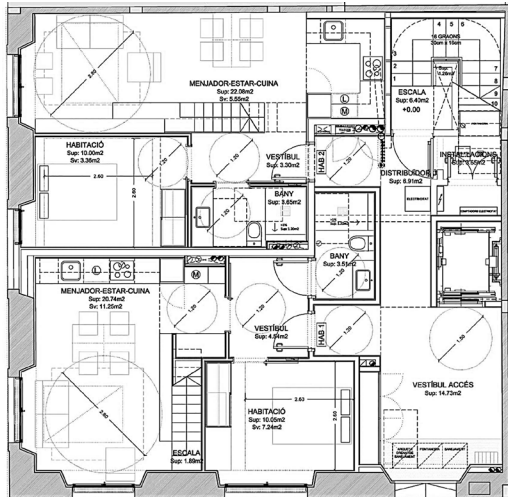
Planta Baja
