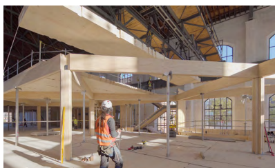
Foto. Rubén Pérez Bescós. Colocación de pieza de forjado -CLT de 13 x 2 m- utilizando el puente grúa.
