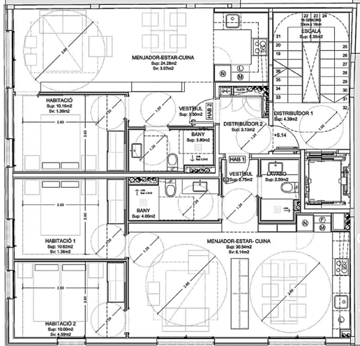
Plantas 1a y 2a
