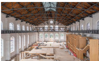
Foto. Rubén Pérez Bescós. Vista del interior de la nave durante el proceso de montaje de la estructura de madera. A la derecha, pantallas estructurales de CLT para los núcleos de ascensores, patinillos y escaleras. Al fondo, puente grúa original del edificio, utilizado para el montaje de la estructura de madera.
