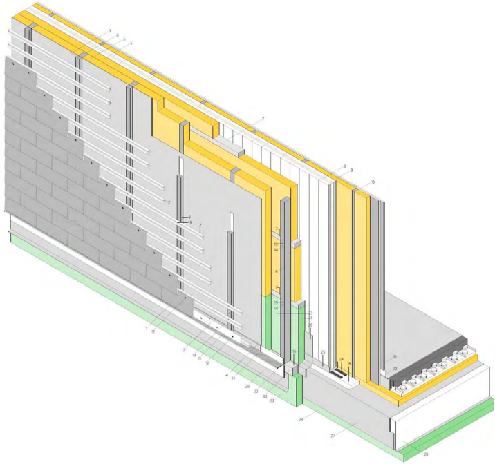
Figura 7: Solución constructiva de fachada.
